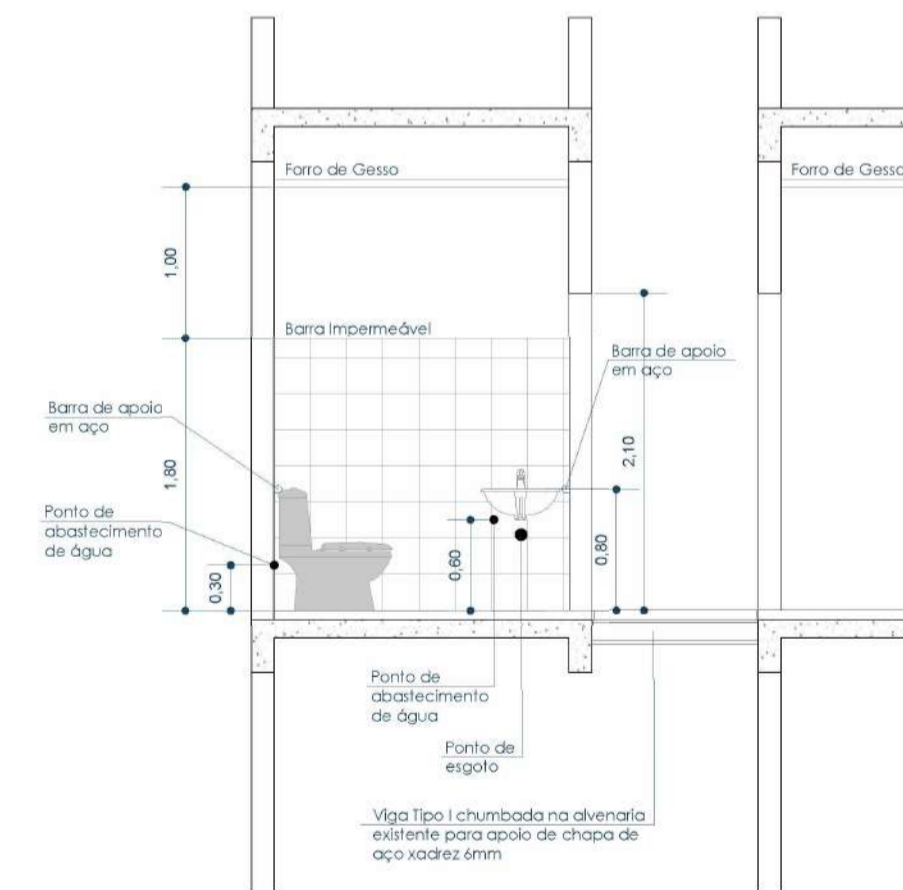
Corte A-A | W.C.PNE Esc. 1 | 50
